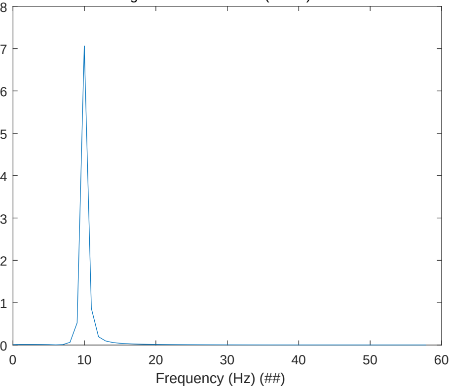
Signal: Sine-Gaussian (##-##)
